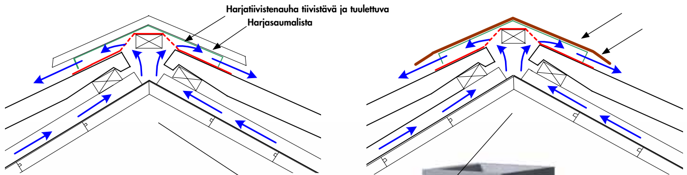
Kuva 1: Rakenne Carisma harjatiilellä
